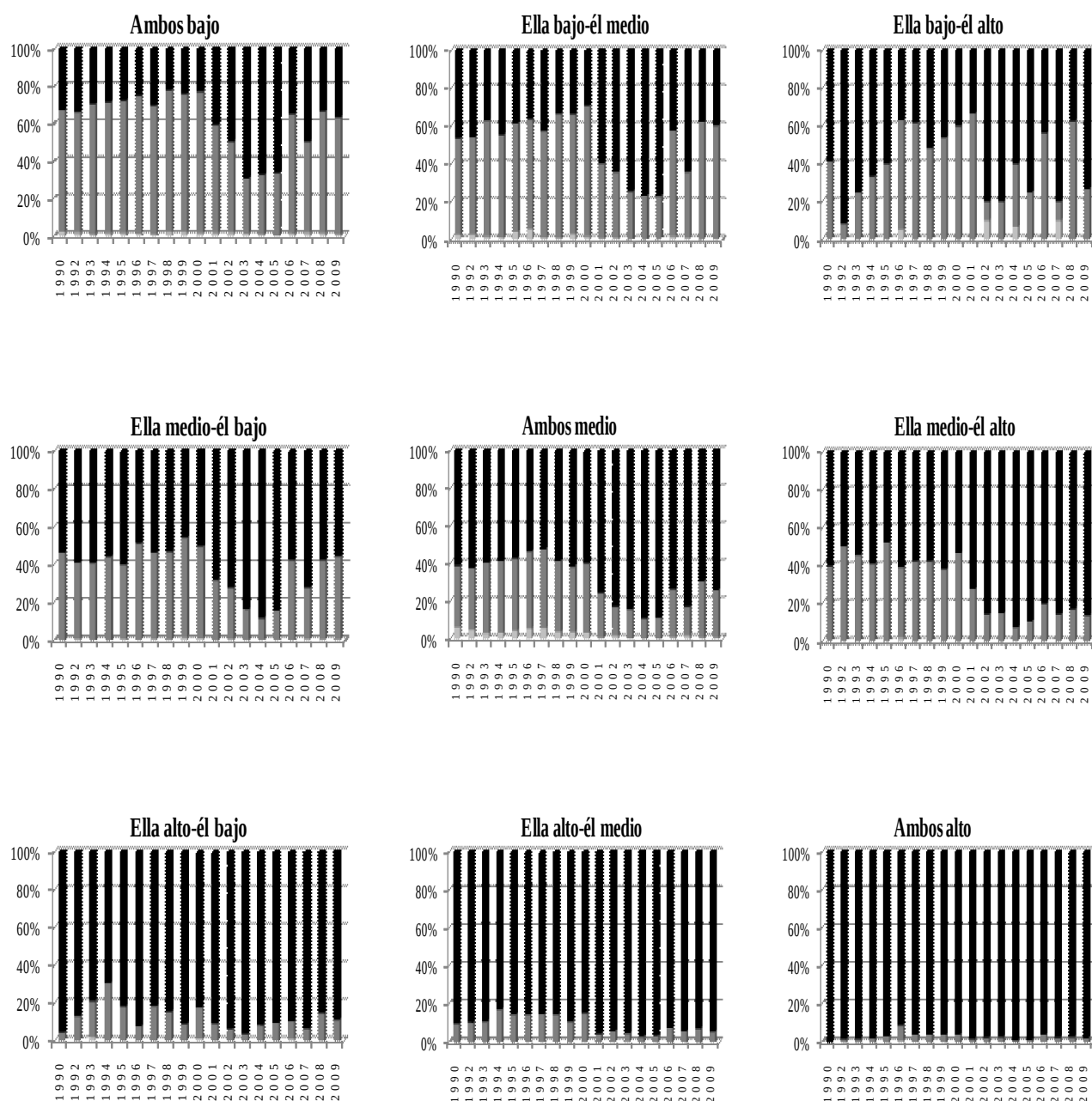
Gráfico 8 : Núcleos según numero de proveedores por capital educativo de la pareja. Rosario 1990-2009
