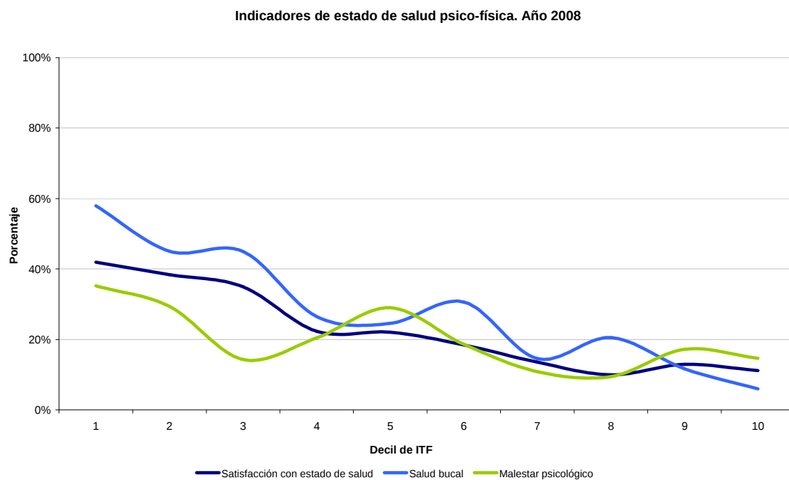
FIGURA 8 y 9: Indicadores de privación en el estado de salud psico-físico según deciles de ITF. Años 2004 y 2008
